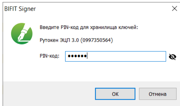
Рис. 18. Ввод PIN-кода
