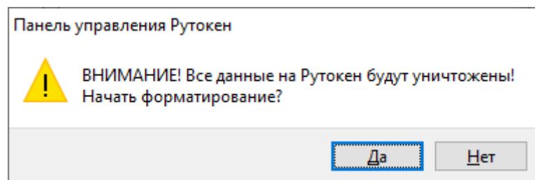
Рис. 27. Предупреждение
